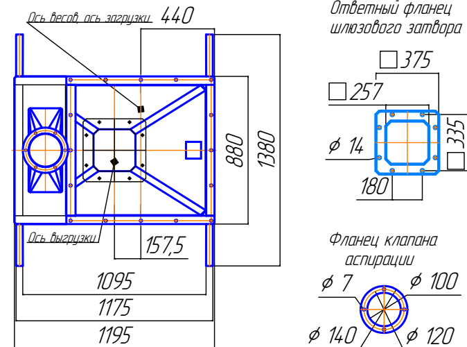
Подвесной бункер вид сверху
