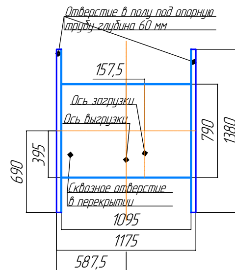
Отверстие в перекрытии под подвесной бункер
