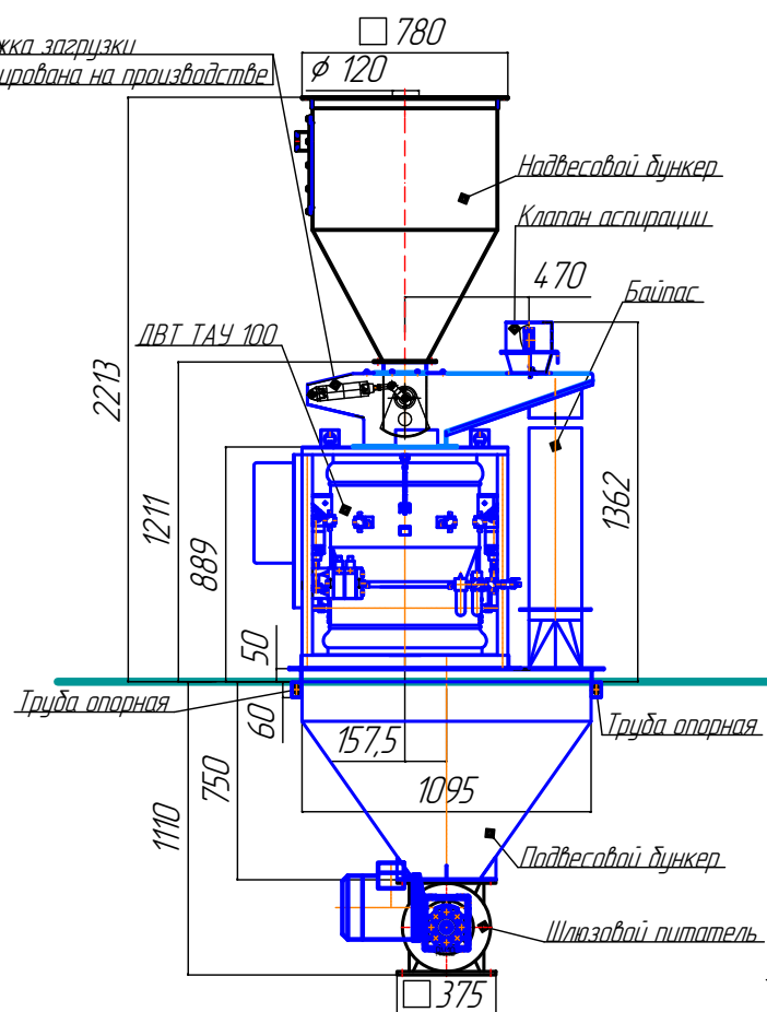
Весы вид спереди
