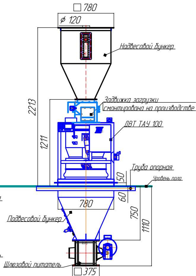
Весы вид слева
